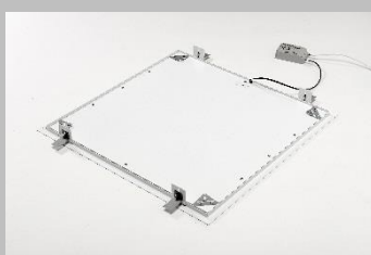
Kit pour montage dans plafonds à découpe
